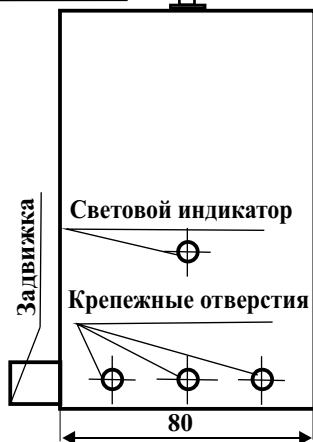
Рис 4 Извещатель пожарный пламени “Пульсар 1-011Н” со снятой розеткой
