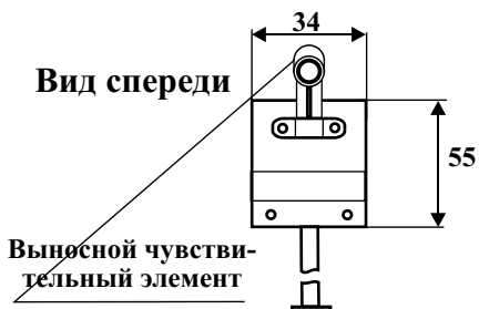
Рис 3 Извещатель пожарный пламени “Пульсар 1-010Н” со снятой розеткой
