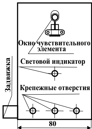
Рис 3 Извещатель пожарный пламени “Пульсар 1-010Н” со снятой розеткой
